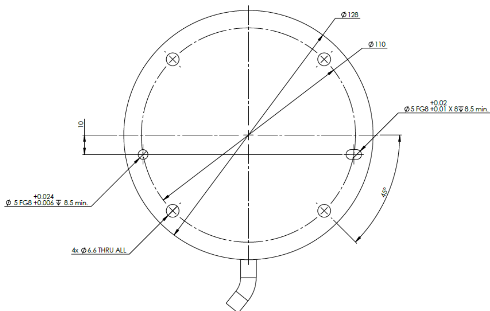
1.1: A robot alapjának alulnézete
